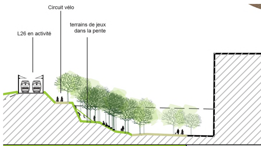
Figure 998: Profil du Parc 26 du site Triangle (ORG 2 , 2018)
